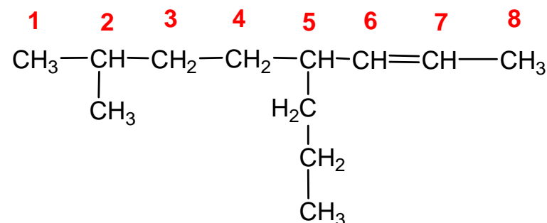
i NO 2-metil-5-propil-6-octè
