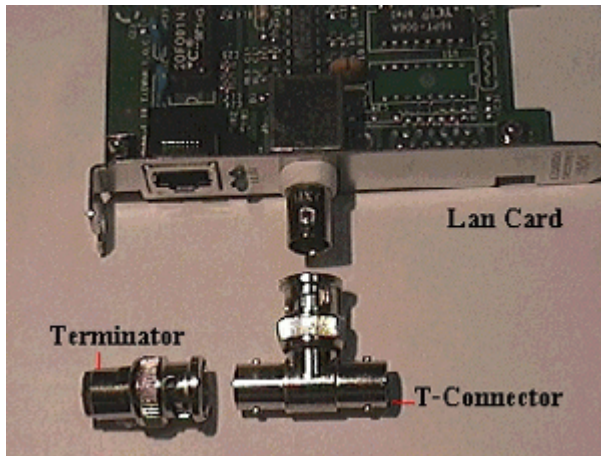
Connector BNC tipus T connectat a targeta de xarxa i terminador
